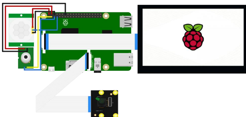
Рис. 1. Структурна схема системи розпізнавання людських образів
