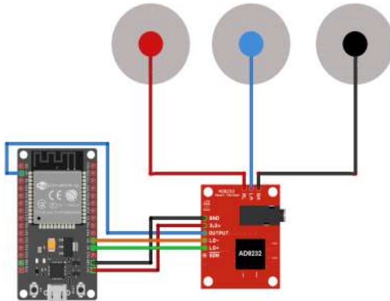
Рис. 2. Блок-схема кардіографа
