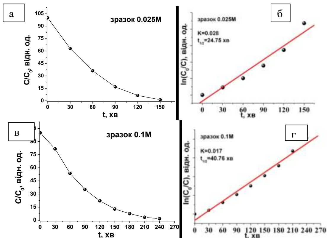
Рис. 1. Залежність концентрації розчину фенолу (а, в) та логарифму відносної зміни концентрації від часу опромінення (б, г) у присутності фотокаталізатора \gamma\text{-Fe}_2\text{O}_3
