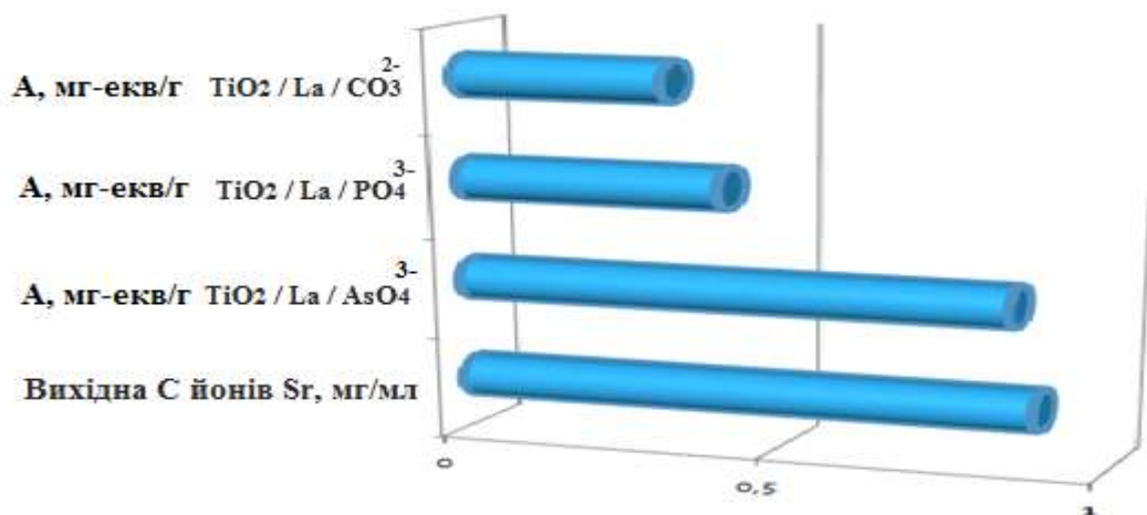
Рис. 1.3. Сорбція йонів Sr із водного розчину \text{SrCl}_2 у нейтральному середовищі адсорбентами на основі сполук Титану
