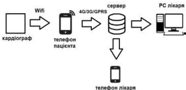
Рис. 1. Структурна схема роботи мережевого кардіографа
